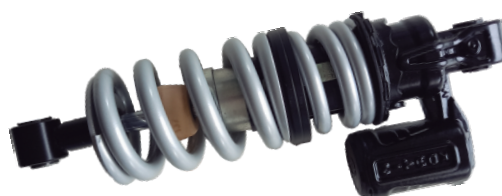
Monoshock - ORIGINAL Cód. 4992 Mola Cinza c/ Regulagem Bajaj Dominar 250
