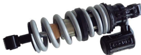
Monoshock - ORIGINAL Cód. 4993 Mola Cinza c/ Regulagem Bajaj Dominar 400 (K10)
